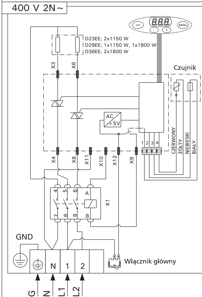
Rys. 12. Schemat elektryczny pieca
