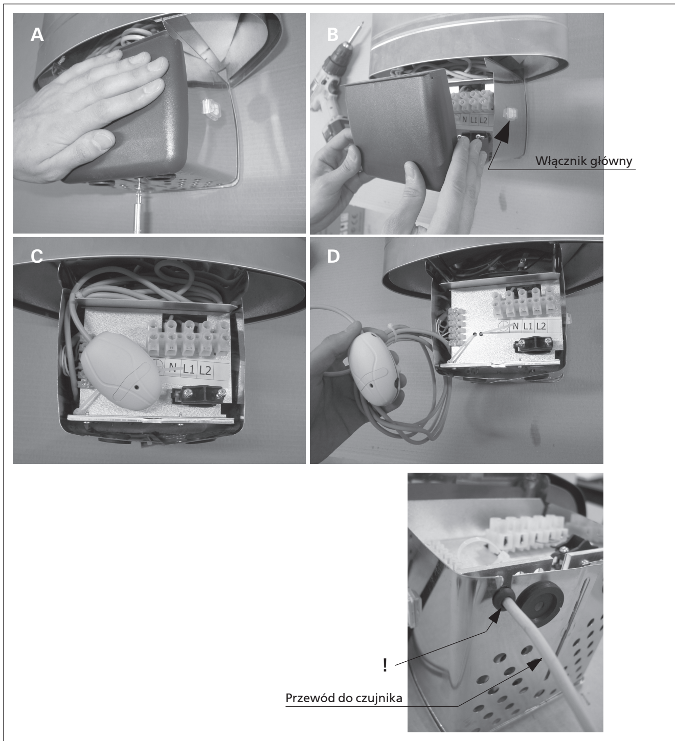
Rys. 10. Otwieranie skrzynki łączeniowej
