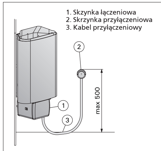
Rys. 8. Kable (wymiary w milimetrach)
