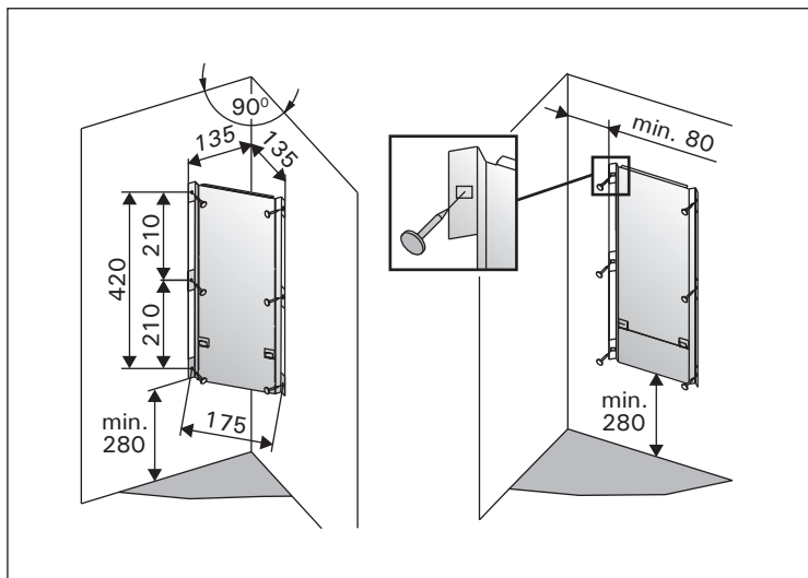
Rys. 7. Usytuowanie wspornika do zawieszenia pieca na ścianie (wymiary w milimetrach)
