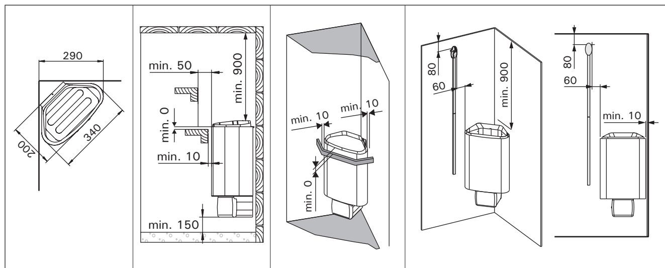
Rys. 6. Minimalne odległości instalacyjne (wymiary w milimetrach)
