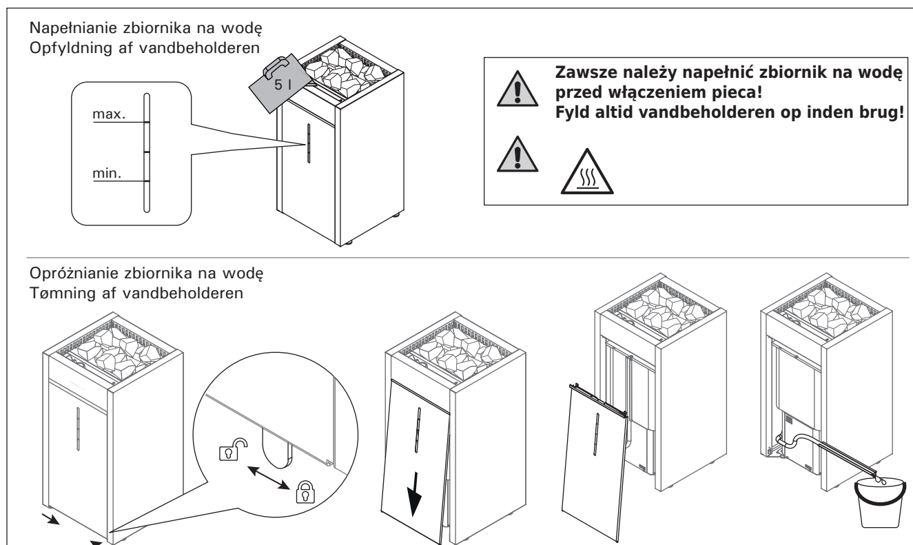
Rys. 2. Napełnianie i opróżnianie zbiornika na wodę
