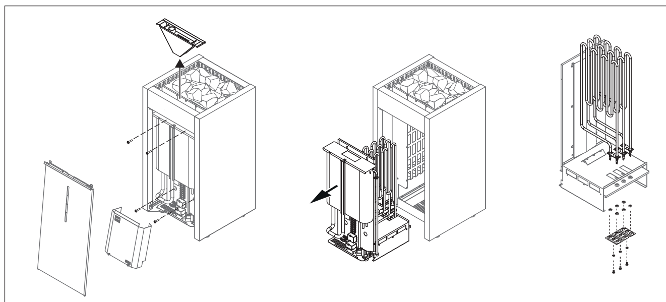
Rys. 11. Wymiana grzałek
