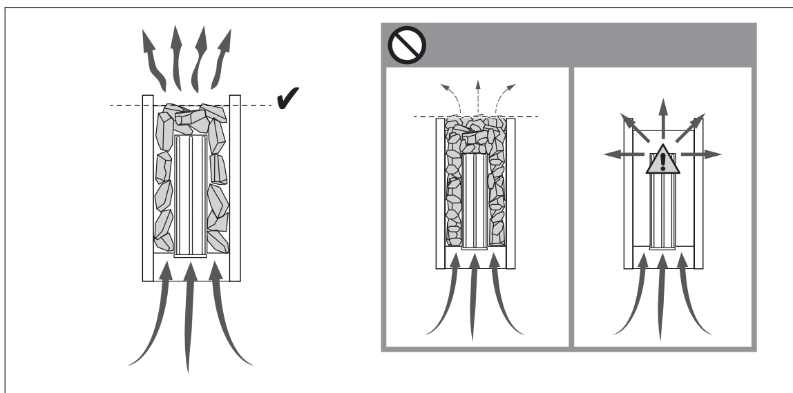
Rys. 1. Układanie kamieni w piecu
