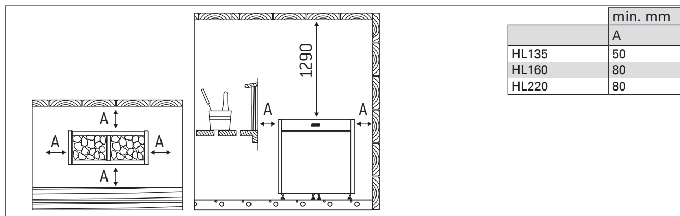
Rys. 4. Minimalne odległości instalacyjne (wymiały w milimetrach)
